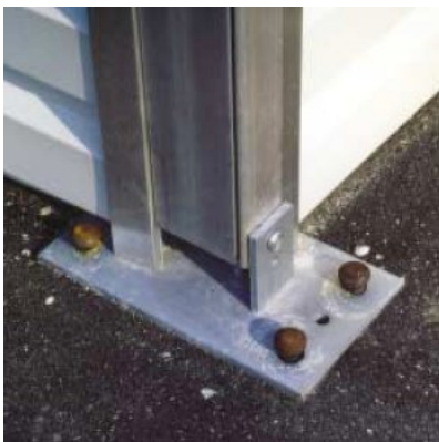
Verankerung mittels Erdnägel
